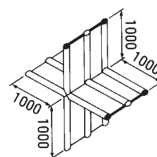
(6)立体クロス (VC)
