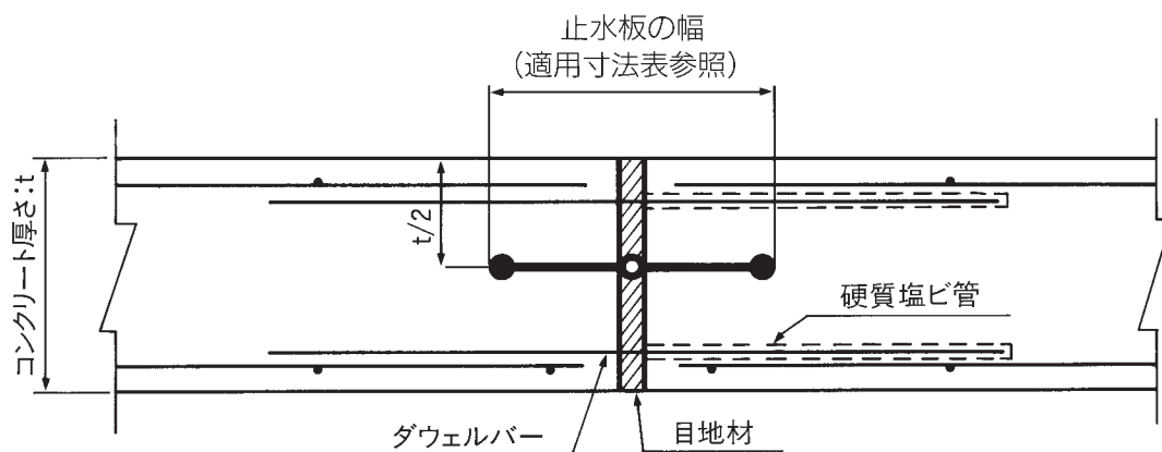
止水板の標準適用寸法
