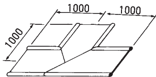
(2)平面チーズ (FT)
