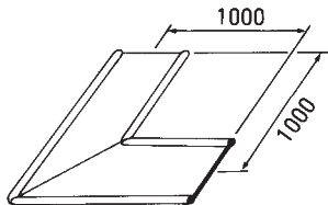
(1)平面エルボ (FL)
