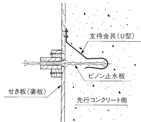
施工例2
