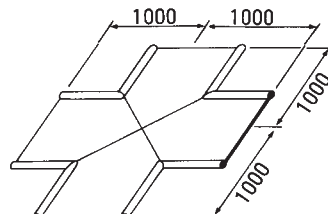
(6)立体クロス (VC)
