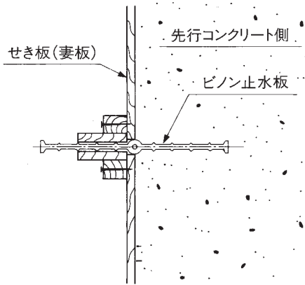
施工例1
