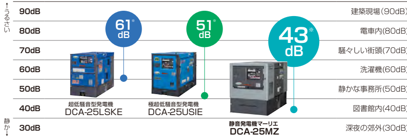
[25kVAクラス発電機 騒音の比較]
