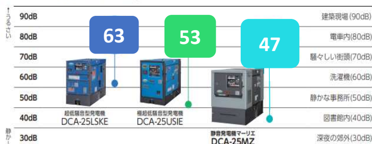
[25kVAクラス発電機 騒音の比較]
