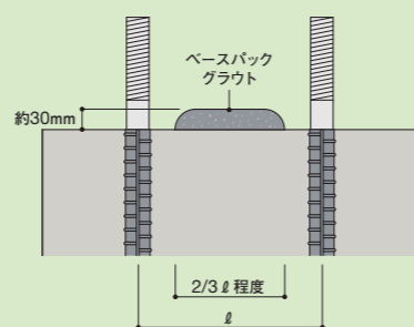
図-1 レベルモルタルの大きさ
