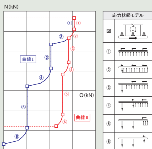
Q-N耐力曲線(柱脚降伏耐力) ※柱脚M-N応力状態により、曲線IIのせん断耐力を用いることができます。
