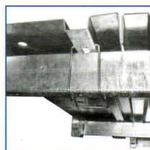
＜クリップ固定式跳ね出し足場＞
