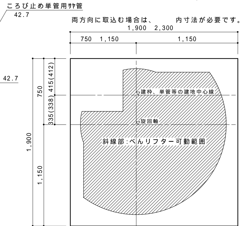
設置必要寸法 S=1/25
