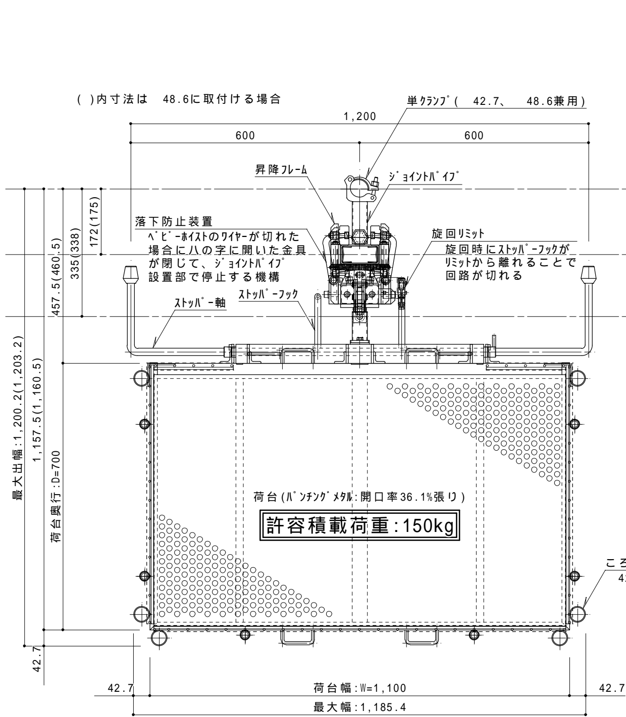
昇降時平面図 S=1/10
