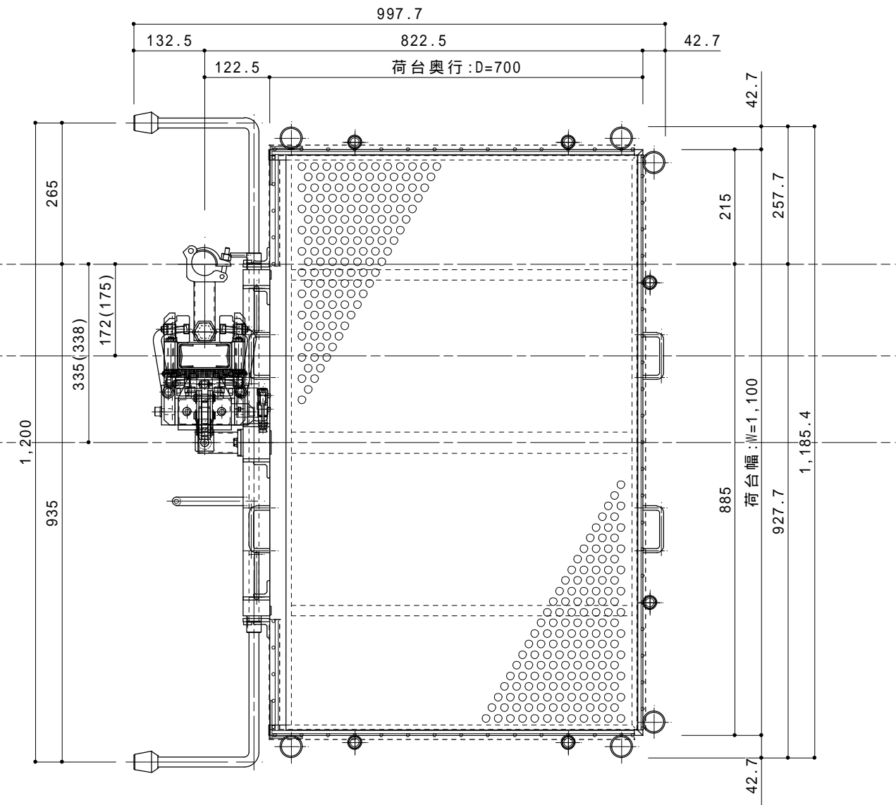
90° 回転時平面図 S=1/10
