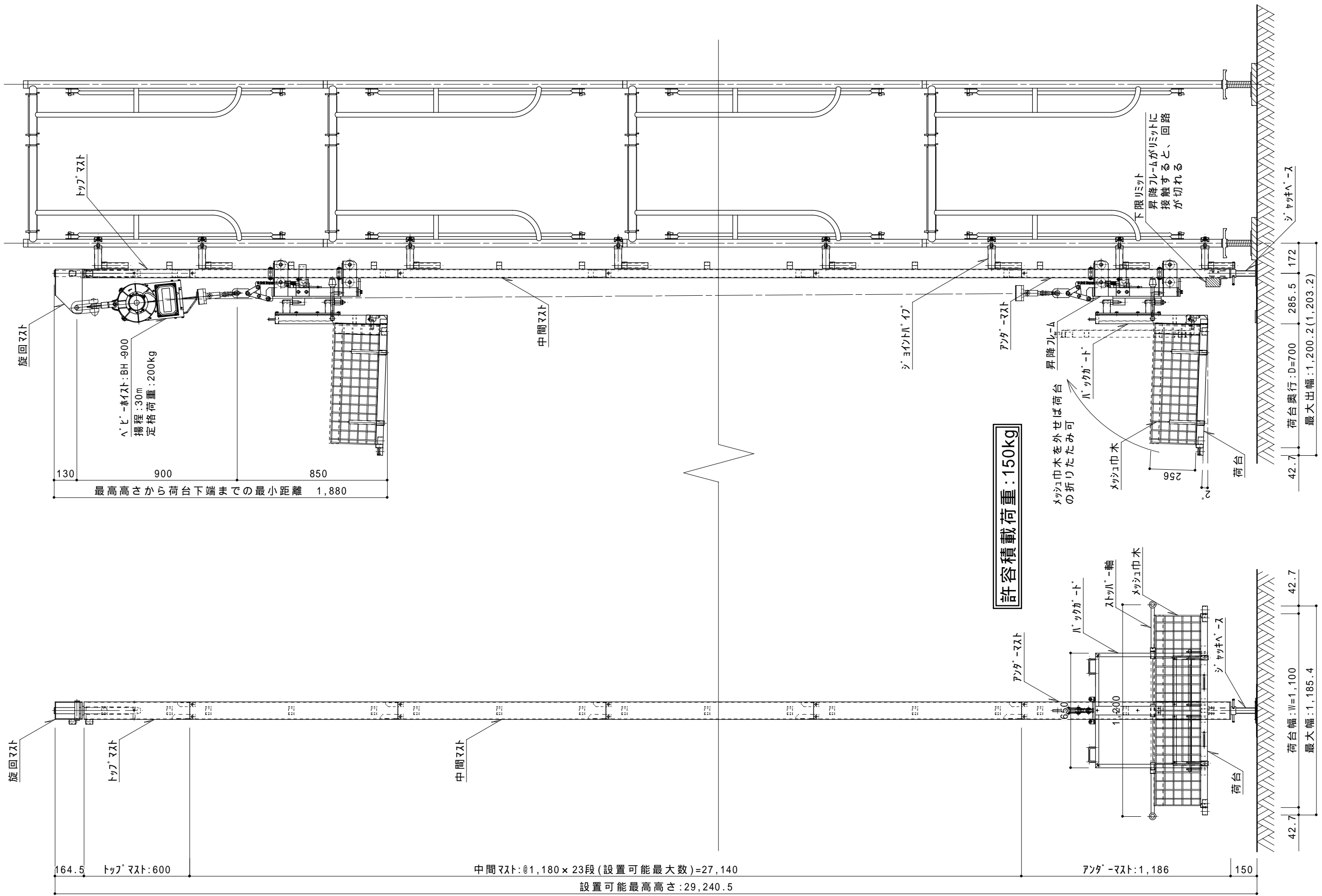
側面図 S=1/20
