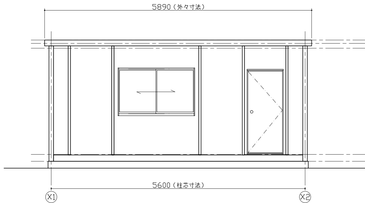
(Y1) 通り立面図
