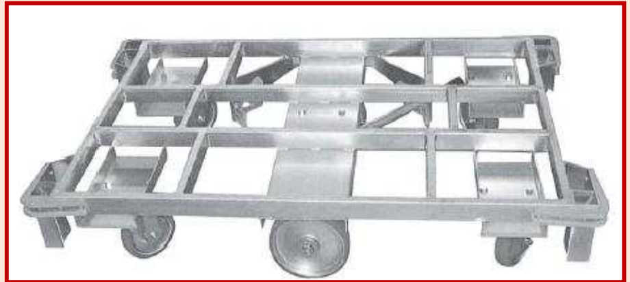
中心の大車輪φ200で段差もスムーズ 初動も移動もラクラク 『六ツゴロウ』
