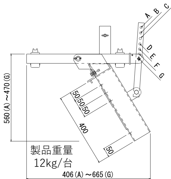
調整角度対応表
