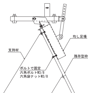
②ボルトで固定する ※ボルト長さは残存型枠の厚みにより変わります
