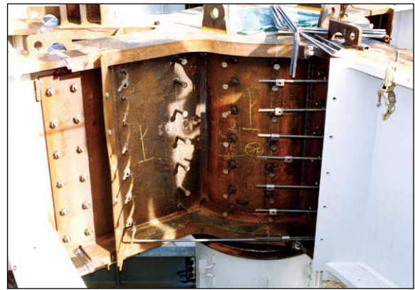
SRC 造仕口部
