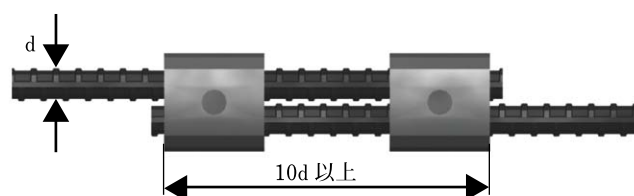
2 個継手【建築】
