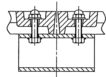
断面 A-B
